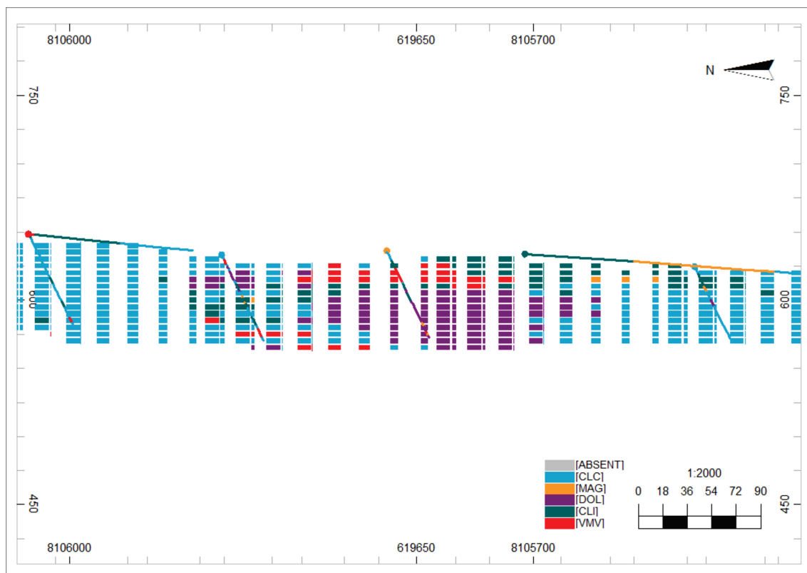
Figura A.4 – Seção transversal C-C'.
