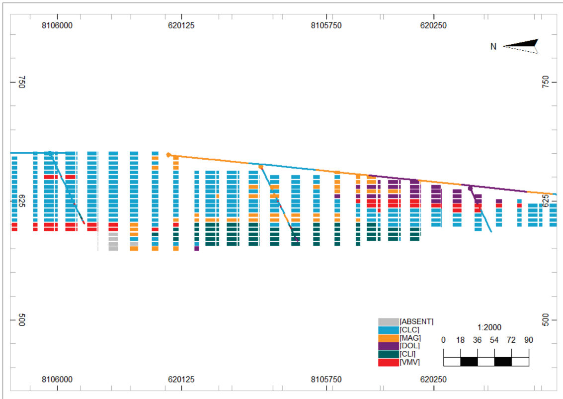
Figura A.6 – Seção transversal E-E'.
