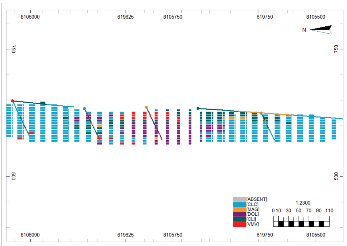
Figura A.3 – Seção transversal B-B'.
