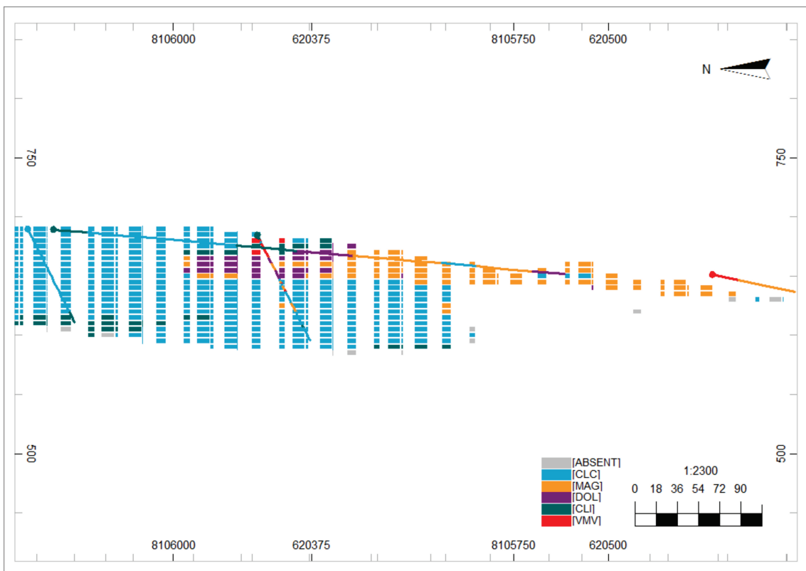
Figura A.7 – Seção transversal F-F'.
