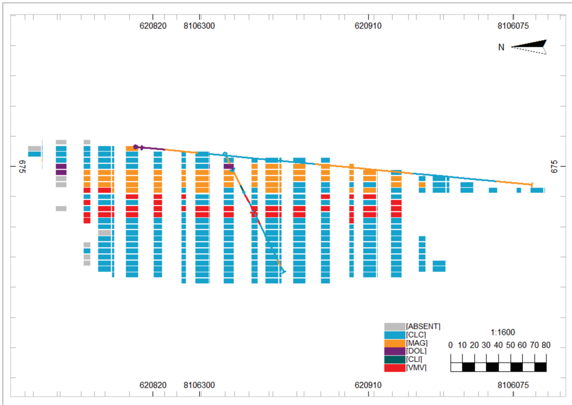
Figura A.2 – Seção transversal A-A'.
