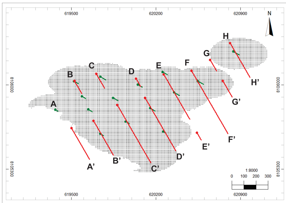
Figura A.1 – Mapa em planta mostrando as posições das seções transversais do modelo geológico.
