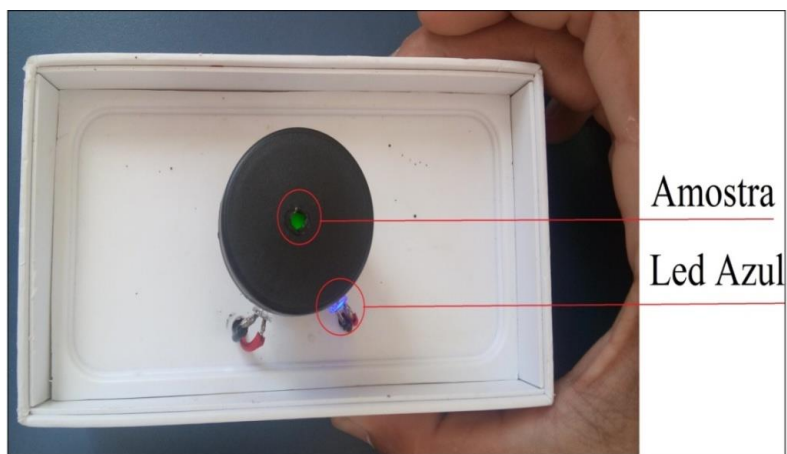
Figura 12 – Experimento montado em uma embalagem de smartphone . Vista superior.
