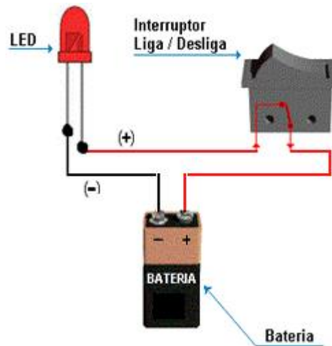
Figura 5 – Esquema elétrico para ligação do LED
