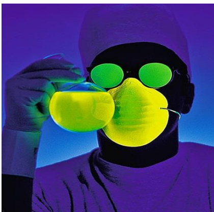
Figura 1 – Materiais com coloração verde fluorescente quando iluminadas com luz adequada.
