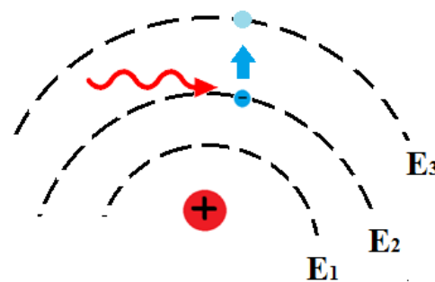
Figura 7 - O elétron “saltará” do nível E_2 para o nível E_3 se absorver um quantum de energia.
