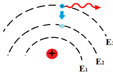
Figura 8 - O elétron retorna do nível de energia E_3 para o nível E_2 , o elétron emite um quantum de energia.
