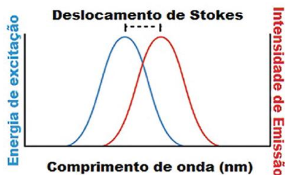
Figura 4 – O deslocamento de Stokes da excitação e emissão em amostras fluorescentes
