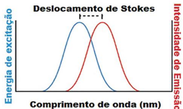
Figura 18 – O deslocamento de Stokes da excitação e emissão em amostras fluorescentes.
