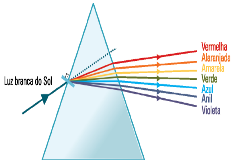
Figura 3 – Decomposição da luz branca
