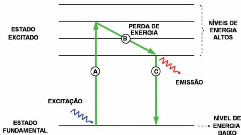
Figura 16 – Diagrama do processo de fluorescência. A – O Elétron salta para um nível de maior energia ao ser estimulado com radiação específica. B – Perda de energia geralmente por vibração molecular e calor. C – Retorno ao estado fundamental com emissão de radiação.
