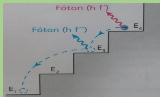
Figura 12—O elétron emite radiação e volta ao nível E_1 de energia por etapas
