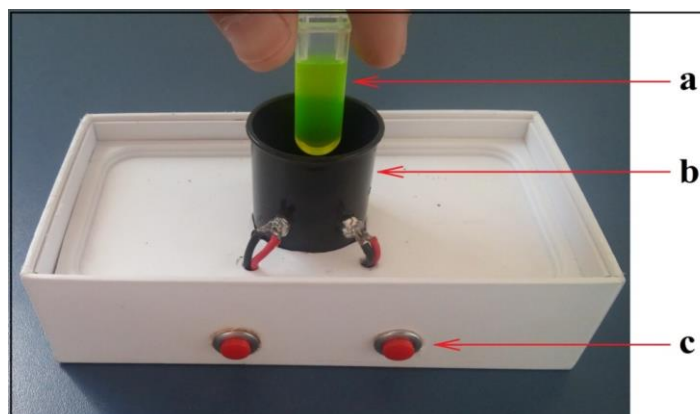
Figura 11 – Experimento montado em uma embalagem de smartphone , a – Porta Amostra com solução, b – Pote de filme fotográfico, c – Botão interruptor.
