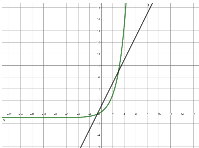
Figura II.3. Função m = 2n + 1 (preto) e função m = 2^n - 1 (verde).
