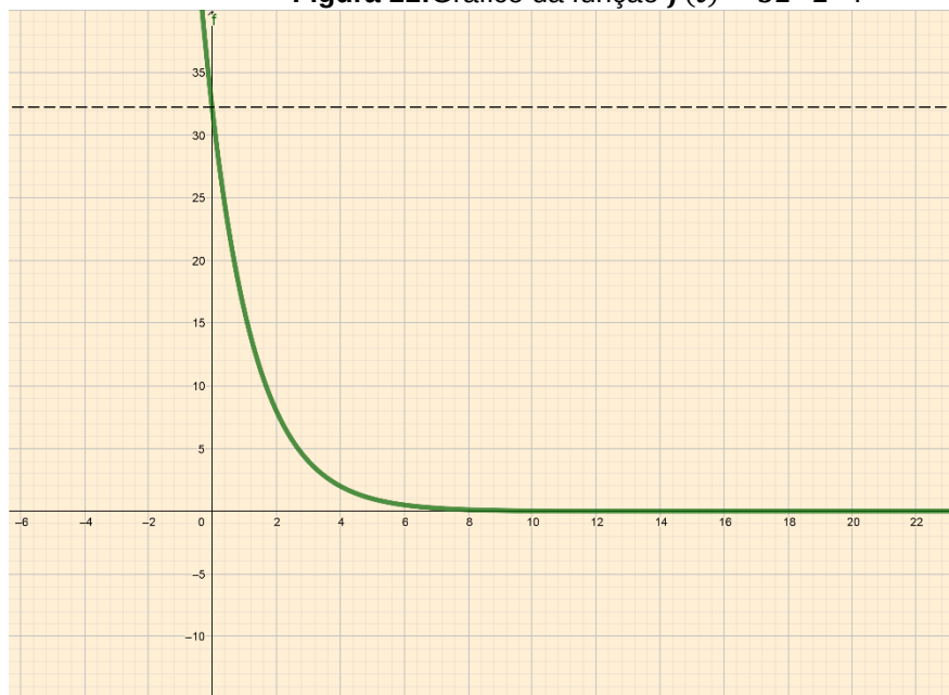
Figura 11: Gráfico da função f(t) = 32 \cdot 2^{-t} .
