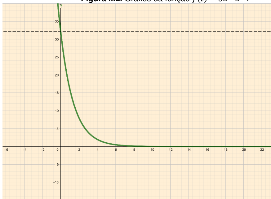
Figura II.2. Gráfico da função f(t) = 32 \cdot 2^{-t} .
