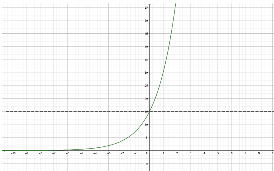
Figura 10: Gráfico da função f(t) = 15 \cdot 2^t
