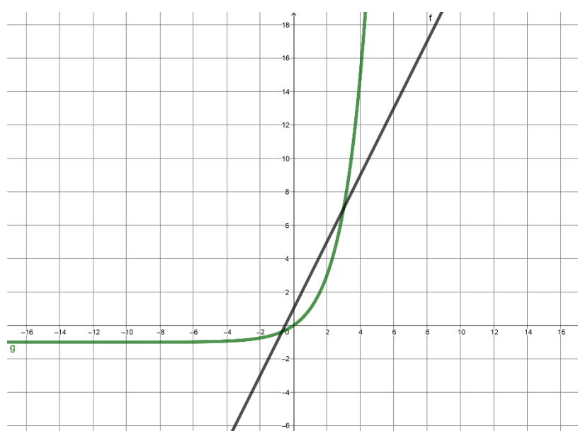
Figura 12: Função m = 2n + 1 (preto) e função m = 2^n - 1 (verde).
