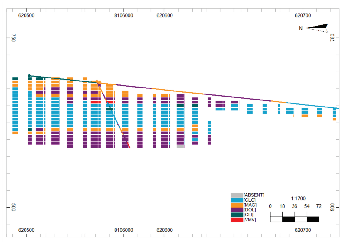
Figura A.8 – Seção transversal G-G'.
