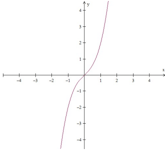
Figura 5: Gráfico da função f(x) = x^3 + x Figura 6: Gráfico da função h(s) = s^3 - s
