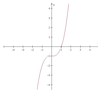
Figura 3: Gráfico da função f(x) = x^3 + 1 Figura 4: Gráfico da função h(s) = s^3 - 1
