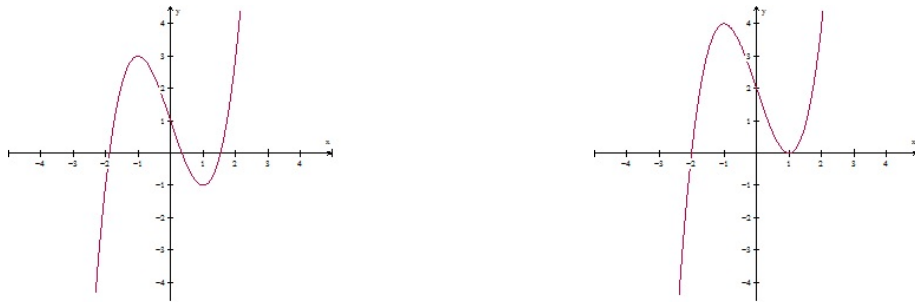
Figura 9: Gráfico da função f(x) = x^3 - 3x + 1 Figura 10: Gráfico da função h(s) = s^3 - 3s + 2
