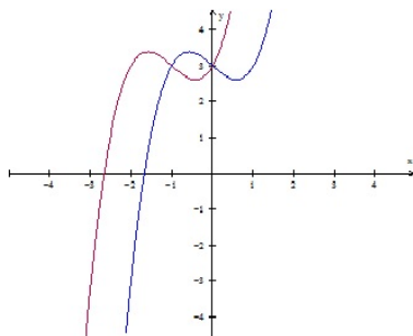
Figura 1: Gráfico das funções f(x) = x^3 + 3x^2 + 2x + 3 e h(s) = s^3 - s + 3
