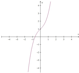
Figura 7: Gráfico da função f(x) = x^3 + x + 1 Figura 8: Gráfico da função h(s) = s^3 - s + 1
