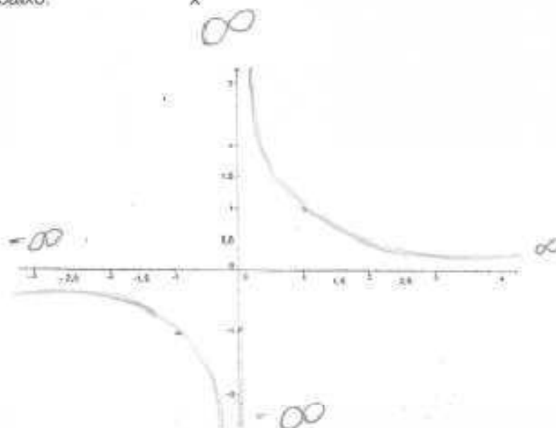
Figura 3: Gráfico de f(x) = \frac{1}{x}
