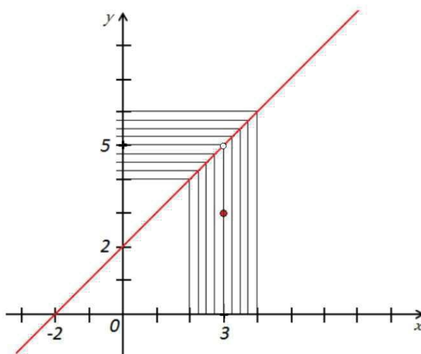
Figura 6: Gráfico de: f(x) = \begin{cases} x+2, & \text{para } x \neq 3 \\ 3, & \text{para } x = 3 \end{cases}
