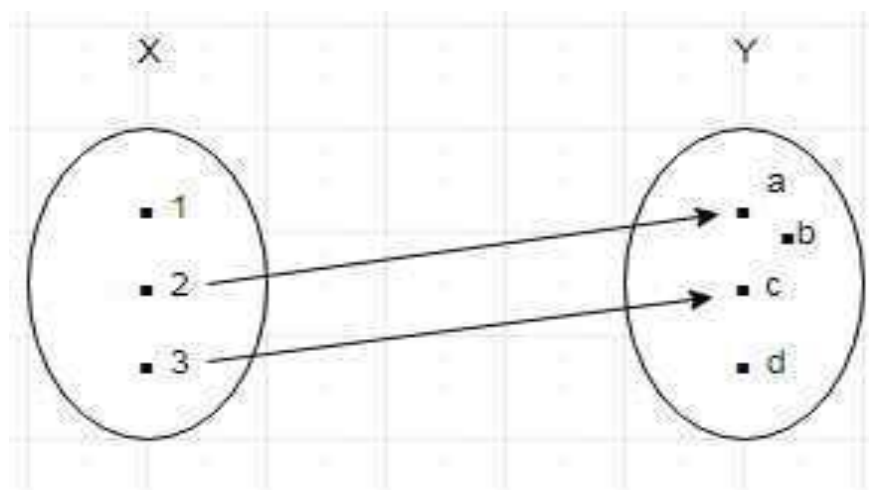
Figura 4: X tem Elementos dos quais não Partem Seta Alguma.
