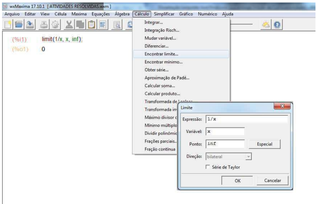
Figura 17: Calculo de Limite no WxMAXIMA com x Tendendo ao Infinito. Fonte: Dados Coletados pelo Autor dessa Pesquisa.
