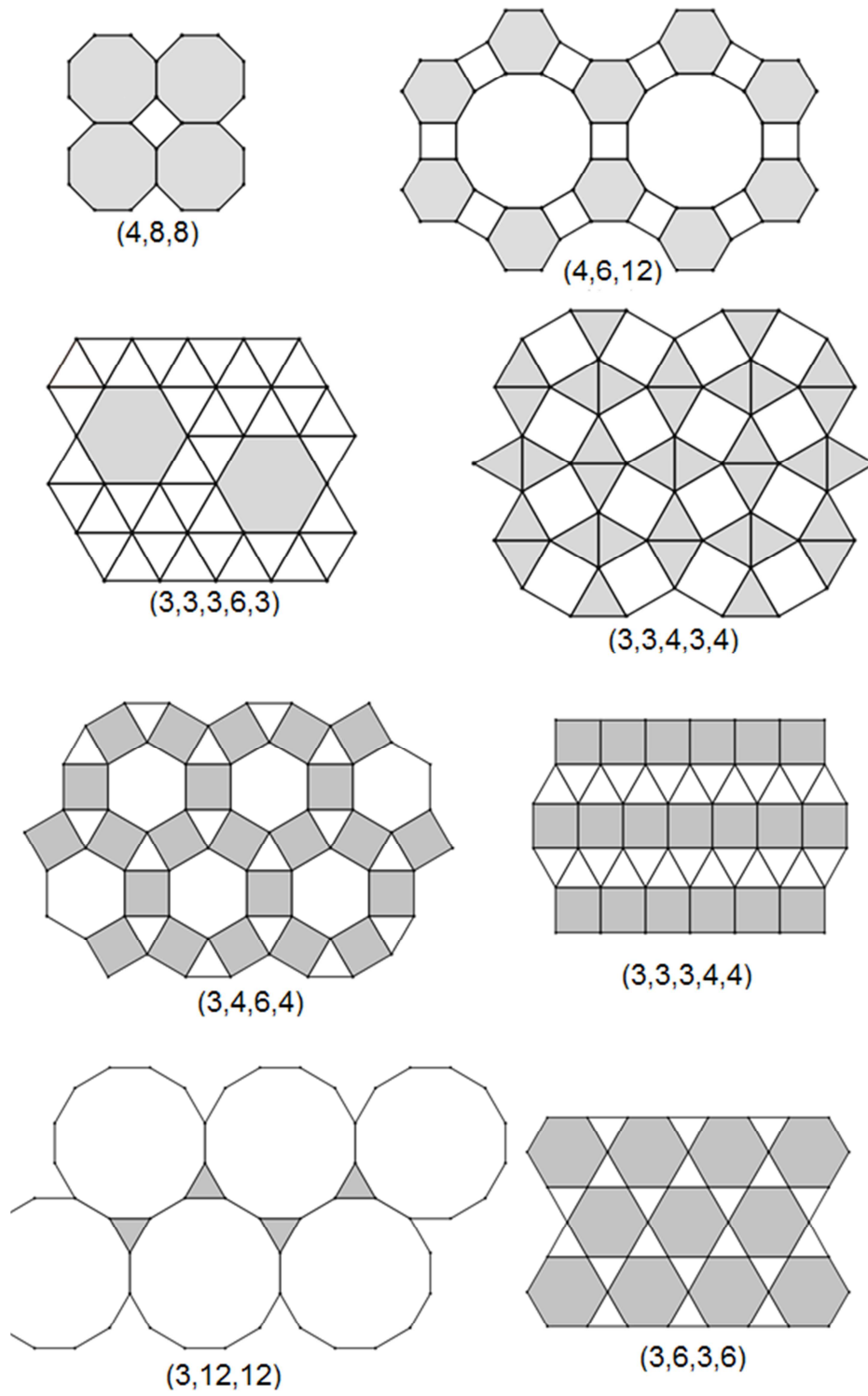
Figura 35: Pavimentações semirregulares.
