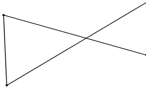
Figura 04: Polígono entrecruzado.
