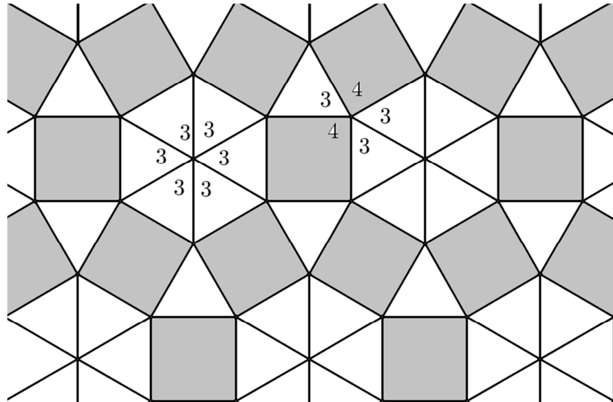
Figura 27: Pavimentação demirregular.
