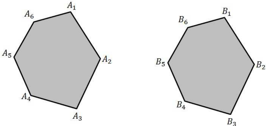
Figura 18: Polígonos congruentes.
