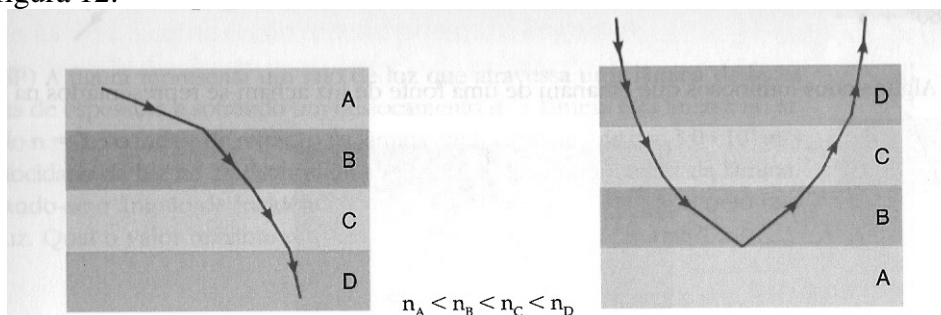
Figura 12 – Lâminas justapostas
