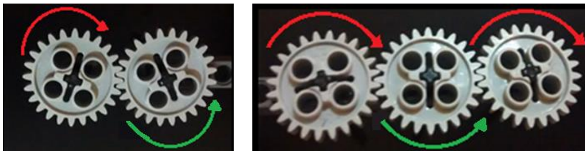
Figura – 13: Orientação dos giros entre as engrenagens motora e movida – Trem Simples.
