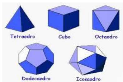
Figura 14. Sólidos platônicos.
